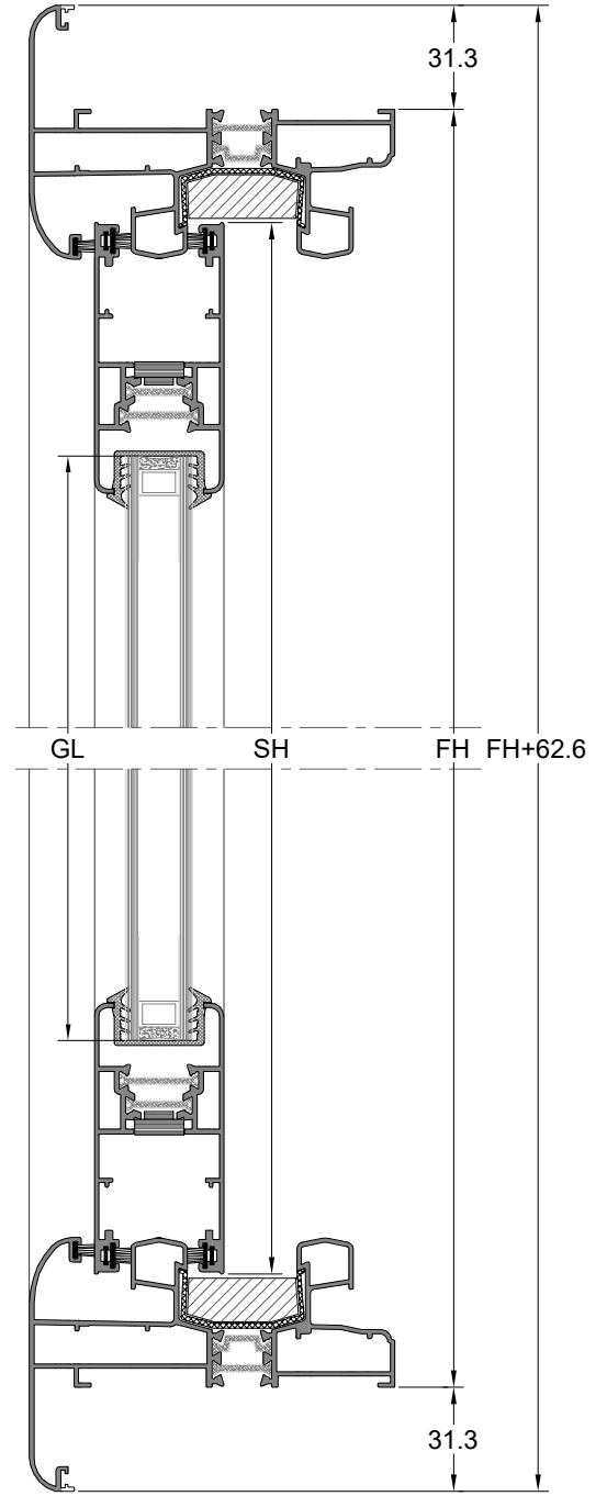
B-B KESİTİ
