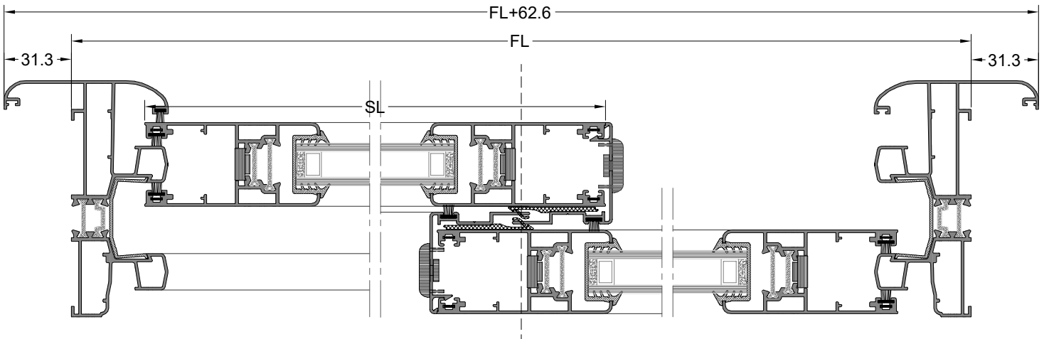
A-A KESİTİ
