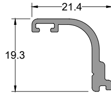
Adaptör Profili (Oval) ADAPTER PROFILE (OVAL)
