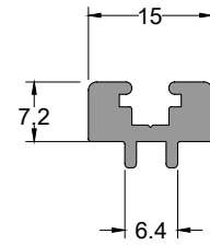
Fırça Adaptörü BRUSH ADAPTER
