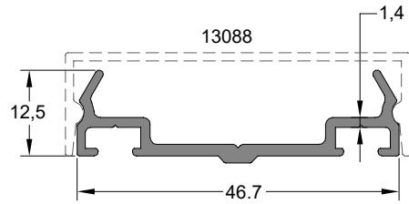
Kapak Altı Baskı Profili COVER UNDER EXTENSION PROFILE
