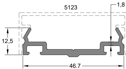
Kapak Altı Baskı Profili COVER UNDER EXTENSION PROFILE
