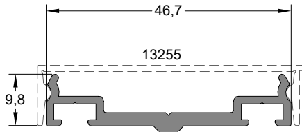
Kapak Altı Baskı Profili COVER UNDER EXTENSION PROFILE
