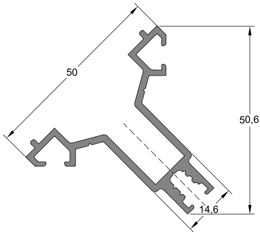
90° Dıştan Köşe Dönüş Adaptör Profili 90° CORNER ADAPTER PROFILE
