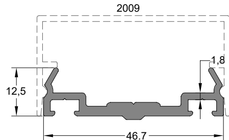
Kapak Altı Baskı Profili COVER UNDER EXTENSION PROFILE
