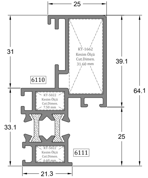
Yalıtımlı Kaset Profili THERMAL BREAK CASSETTE PROFILE
