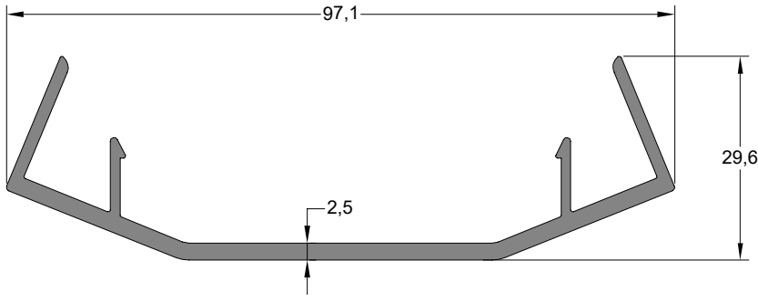
135° Köşe Dönüş Profili 135° CORNER COVER PROFILE
