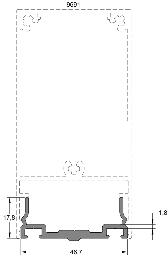
Kapak Altı Baskı Profili COVER UNDER EXTENSION PROFILE
