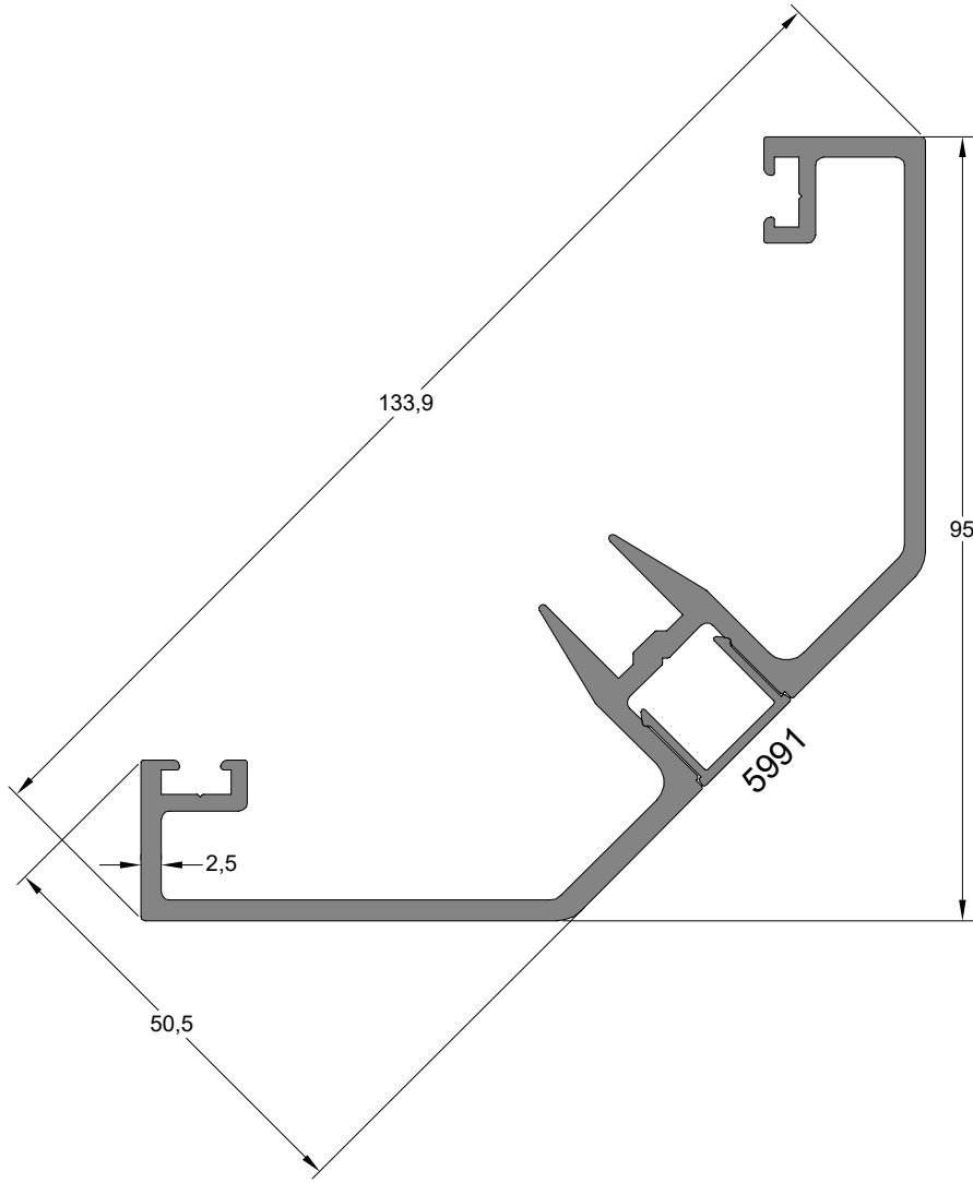
90° Dıştan Köşe Dönüş Kapak Profili 90° CORNER COVER PROFILE
