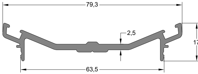
135° Köşe Dönüş Baskı Profili 135° CORNER EXTENSION PROFILE
