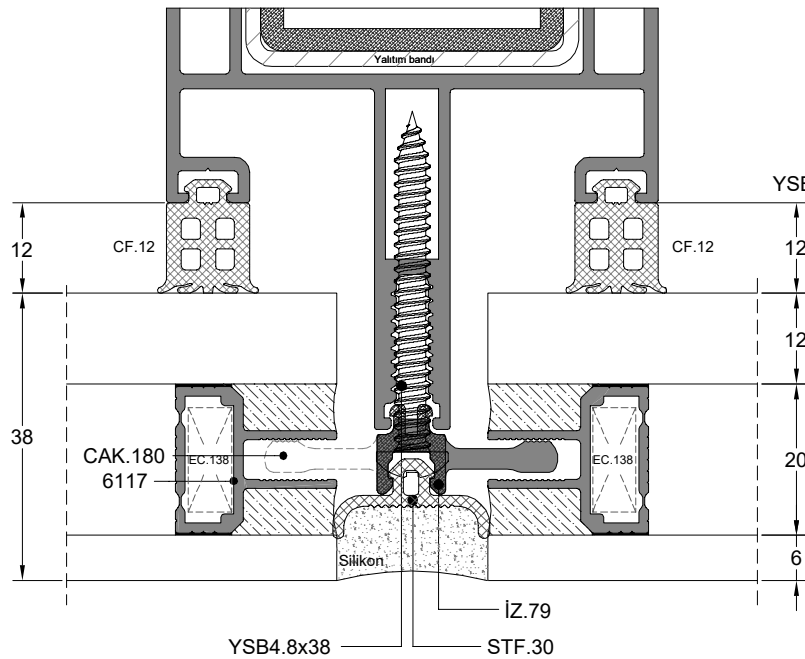
DÜŞEY DETAYI VERTICAL DETAIL
