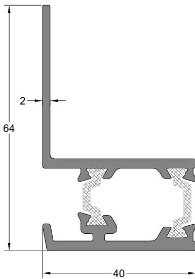
Duvar Bitiş Profili WALL FINISH PROFILE
