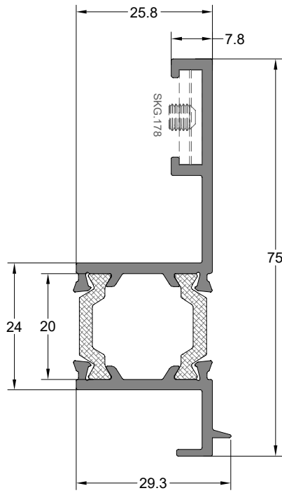
Geçiş Adaptör Profili TRANSITION ADAPTER PROFILE
