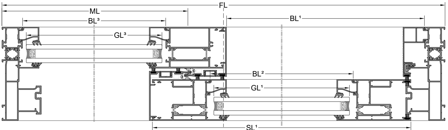
A-A KESİTİ
