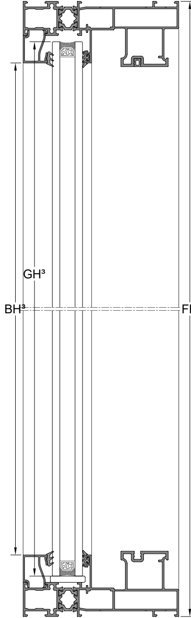
B-B KESİTİ
