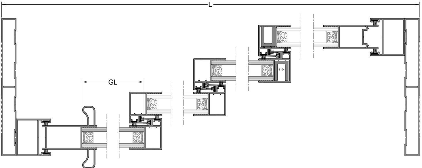
A-A KESİTİ
