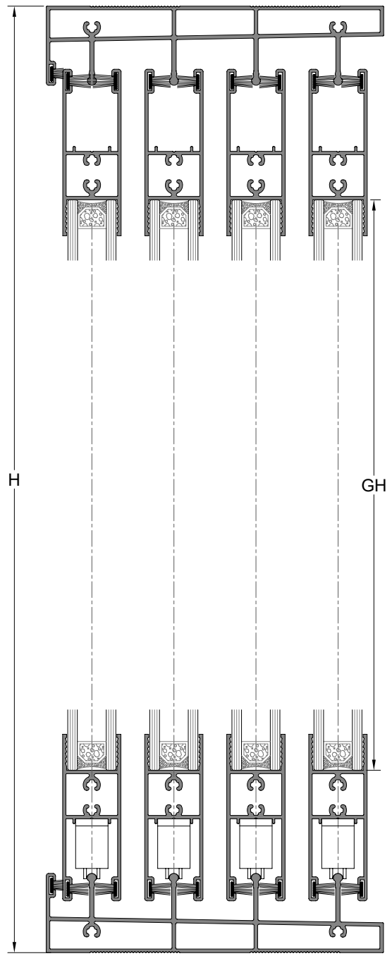
B-B KESİTİ
