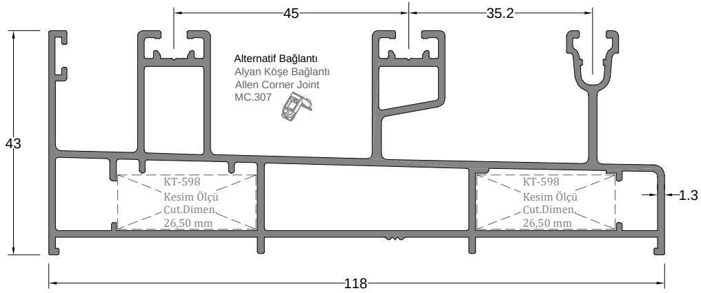
İki Raylı Sineklikli Kasa Profili DOUBLE RAIL SCREENING FRAME PROFILE
