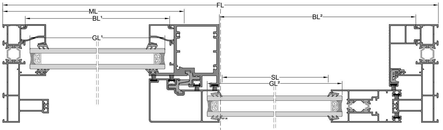
A-A KESİTİ
