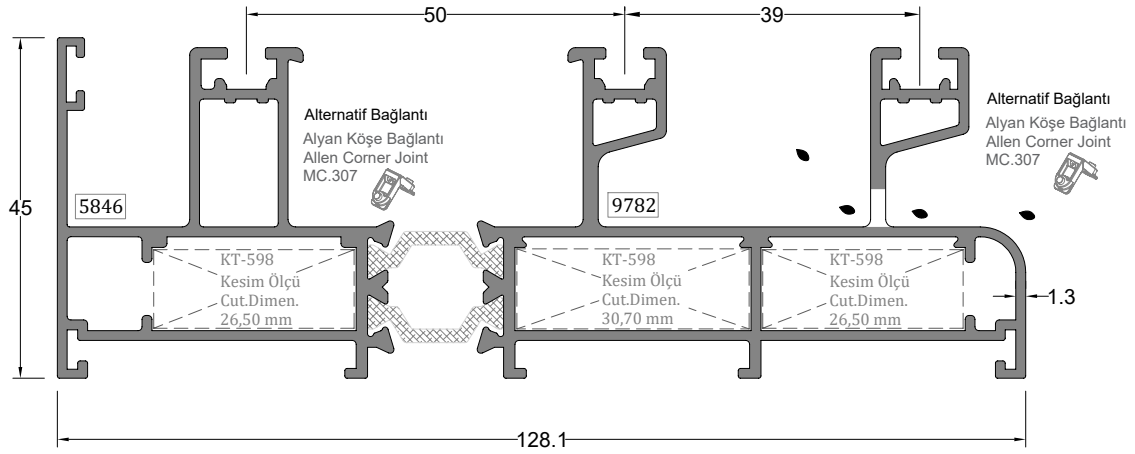
İki Raylı Sineklikli Kasa Profili DOUBLE RAIL SCREENING FRAME PROFILE
