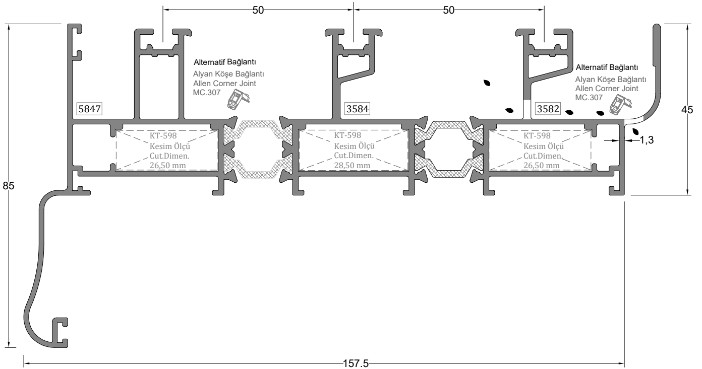
Üç Raylı Sineklikli Kasa Profili TRIPLE RAIL SCREENING FRAME PROFILE
