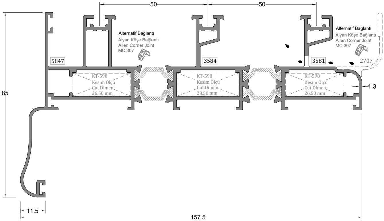
Üç Raylı Sineklikli Kasa Profili TRIPLE RAIL SCREENING FRAME PROFILE
