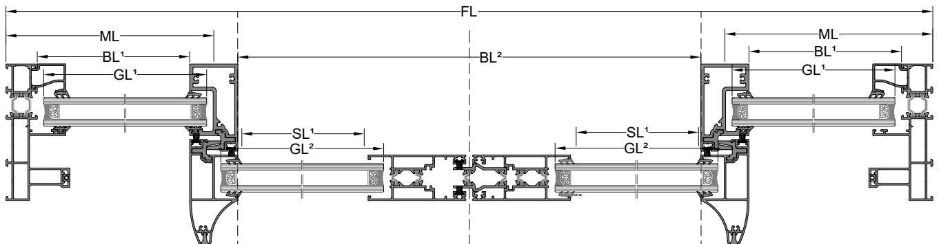
A-A KESİTİ
