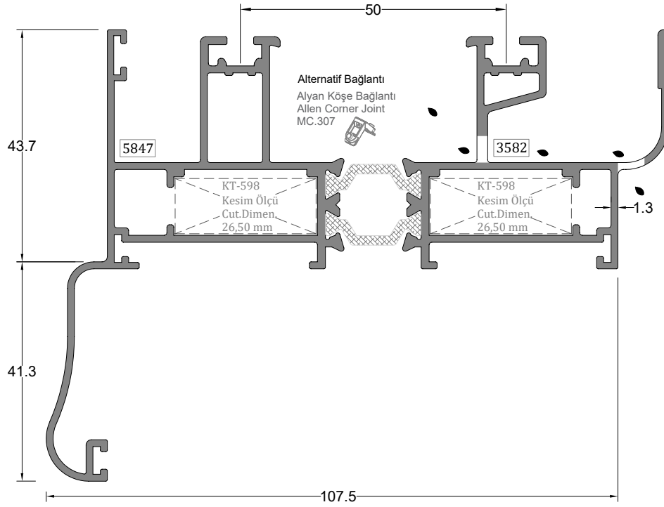
İki Raylı Sineklikli Kasa Profili DOUBLE RAIL SCREENING FRAME PROFILE
