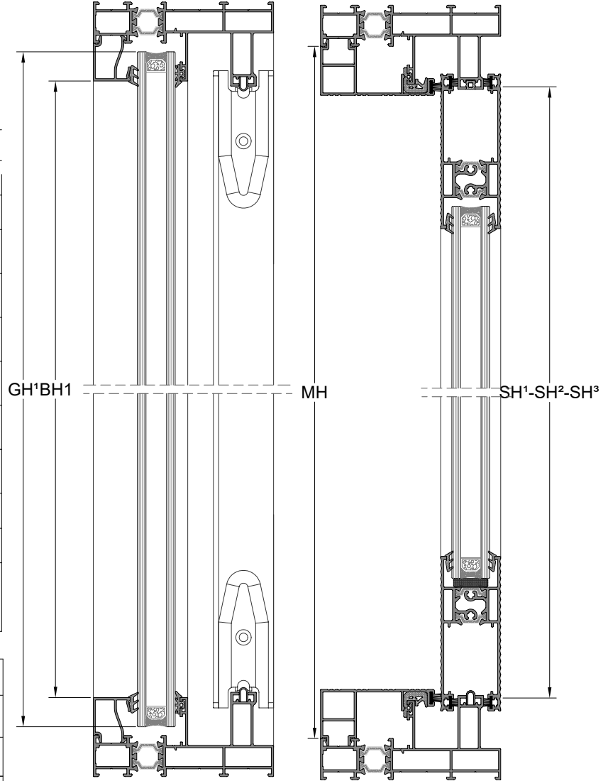
C-C KESİTİ
