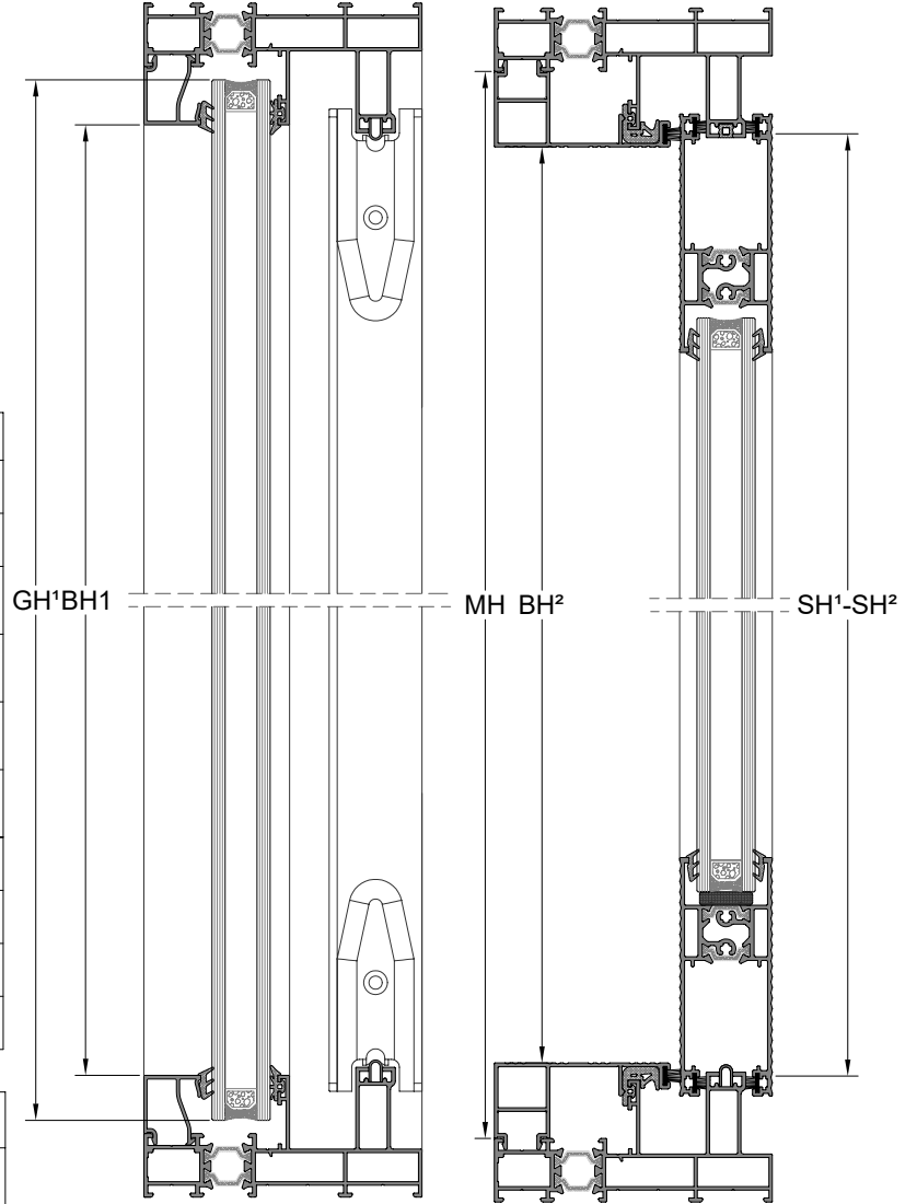
C-C KESİTİ
