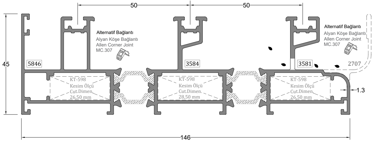
Üç Raylı Kasa Profili TRIPLE RAIL FRAME PROFILE
