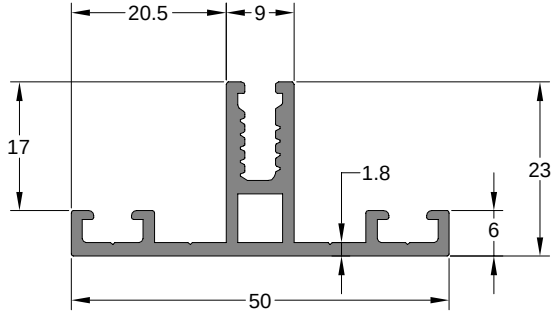
Düşey-Yatay Taşıyıcı Profili VERTICAL-HORIZONTAL CARRIER PROFILE
