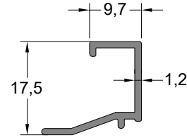
Sineklik Çita Profili SCREENING BEAD PROFILE
