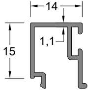
Çita Profili BEAD PROFILE
