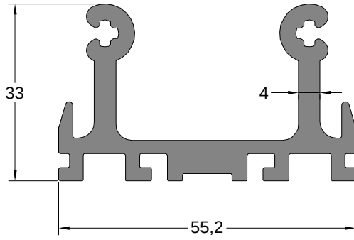
Dik Bağlantı Profili CONNECTION PROFILE
