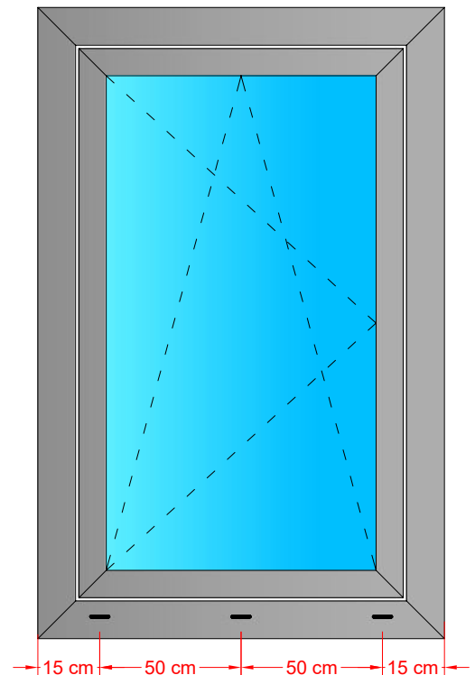
Su Tahliye Delikleri
