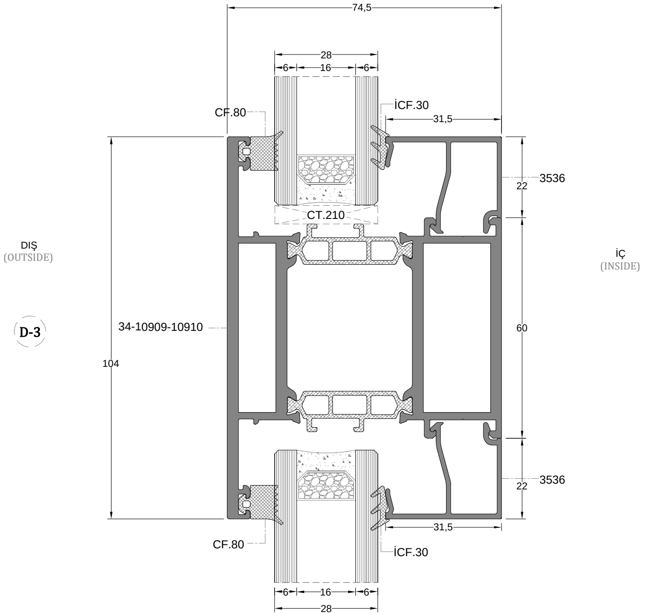
HEMYÜZ DIŞA AÇILIR KAPI DETAY
