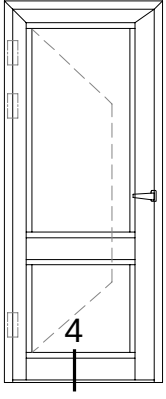
HEMYÜZ DIŞA AÇILIR KAPI DETAY
