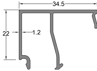
Çita Profili BEAD PROFILE
