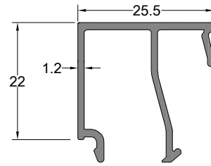
Çita Profili BEAD PROFILE
