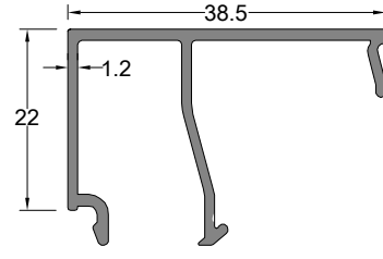
Çita Profili BEAD PROFILE
