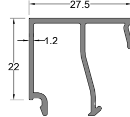
Çita Profili BEAD PROFILE
