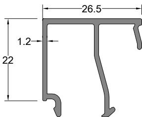
Çita Profili BEAD PROFILE
