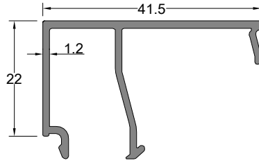
Çita Profili BEAD PROFILE
