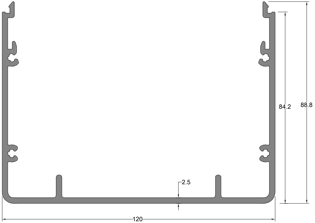
Gider Gizleme Profili DRAINAGE CONCEALING PROFILE
