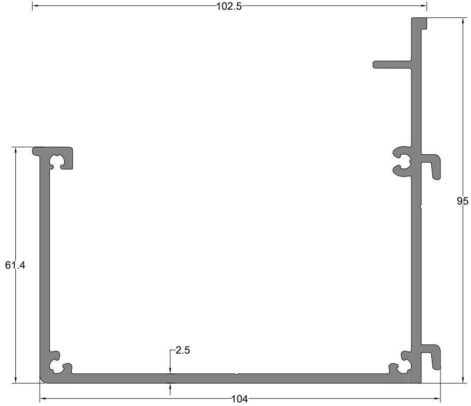
Oluk Profili GUTTER PROFILE
